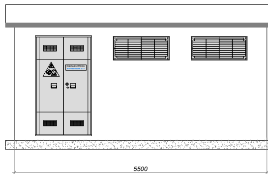
PROSPETTO A
