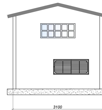
PROSPETTO D
