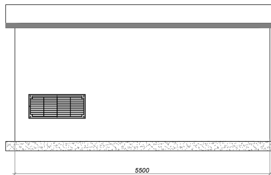
PROSPETTO C
