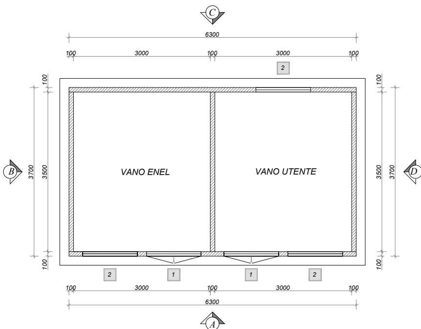
PIANTA CABINA A PANNELLI
