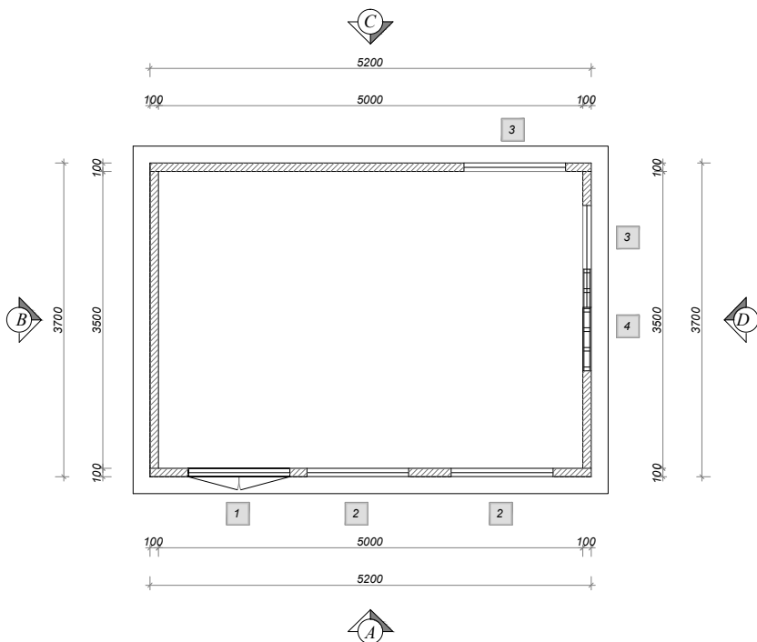
PIANTA CABINA A PANNELLI
