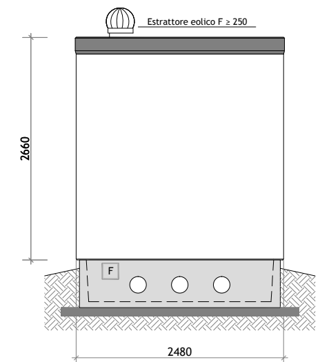
PROSPETTO D
