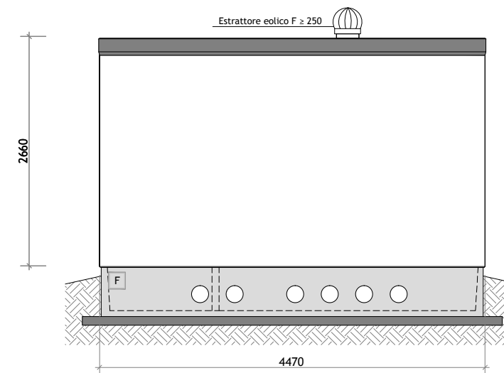
PROSPETTO C
