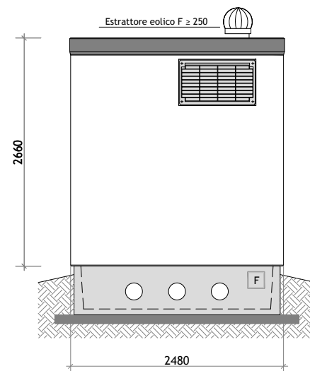
PROSPETTO B
