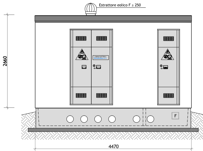
PROSPETTO A
