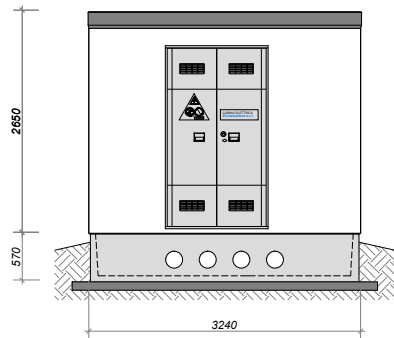
PROSPETTO A
