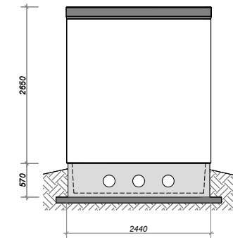
PROSPETTO D
