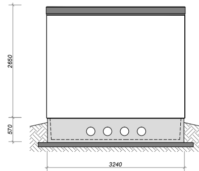
PROSPETTO C
