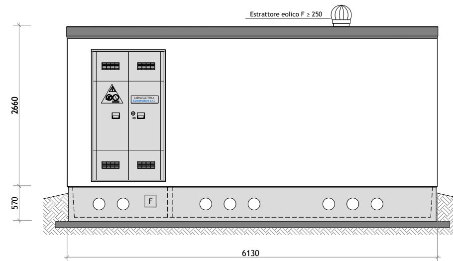
PROSPETTO C
