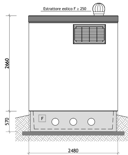
PROSPETTO B
