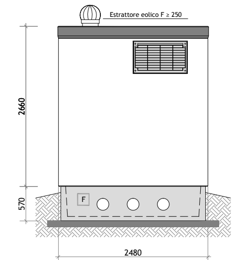
PROSPETTO D
