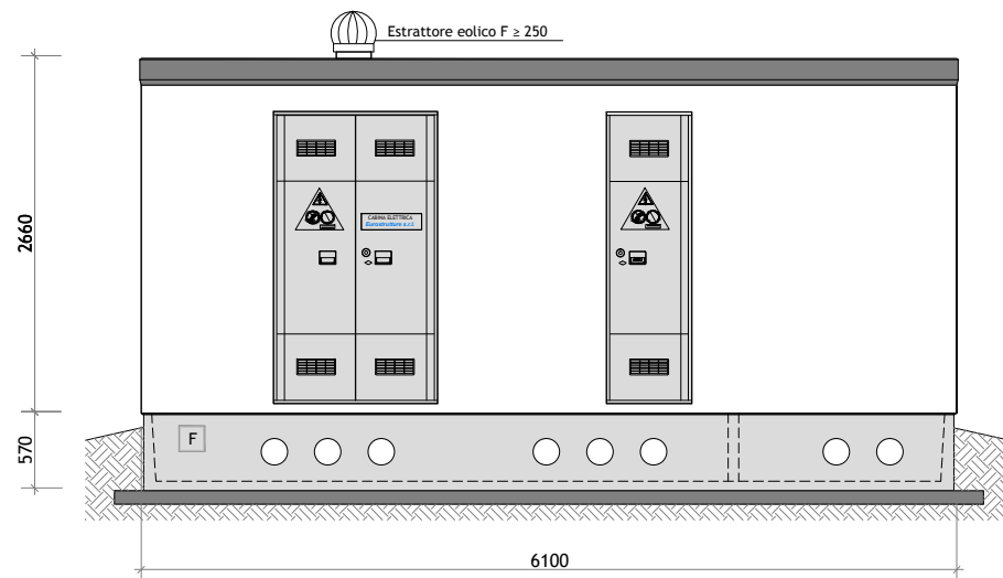
PROSPETTO A
