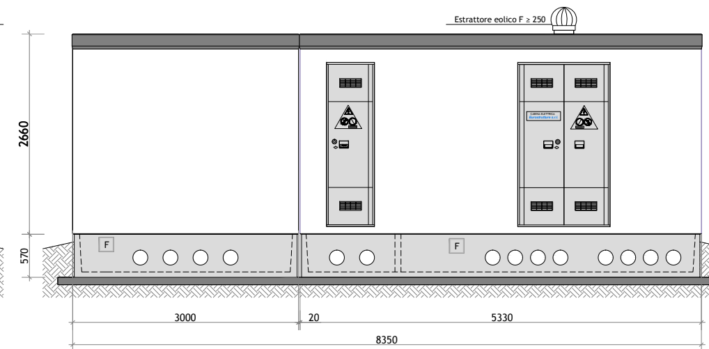
PROSPETTO C
