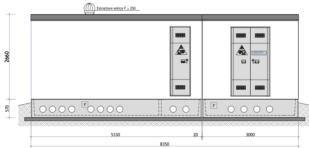
PROSPETTO A
