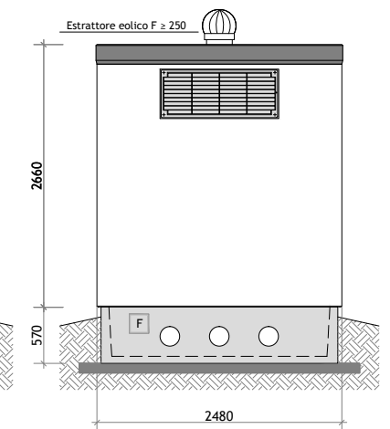
PROSPETTO D
