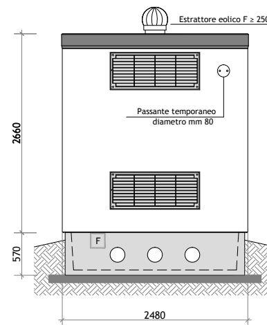
PROSPETTO B
