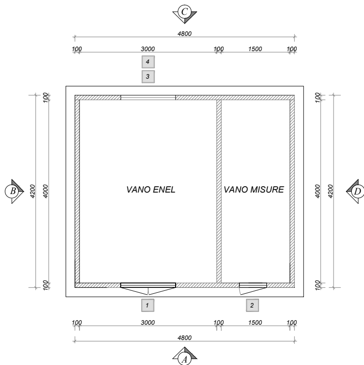
PIANTA CABINA A PANNELLI
