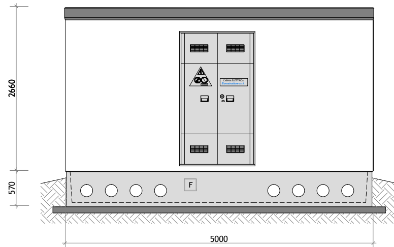
PROSPETTO A
