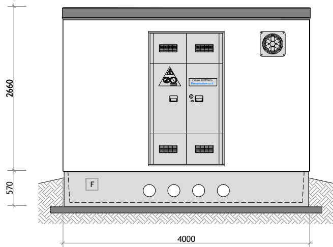
PROSPETTO A
