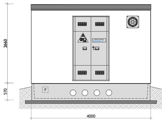
PROSPETTO A
