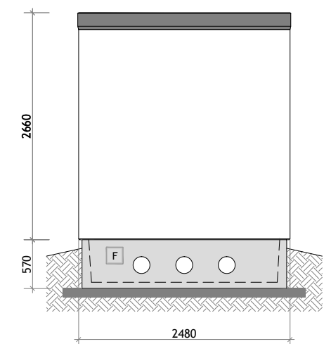
PROSPETTO D
