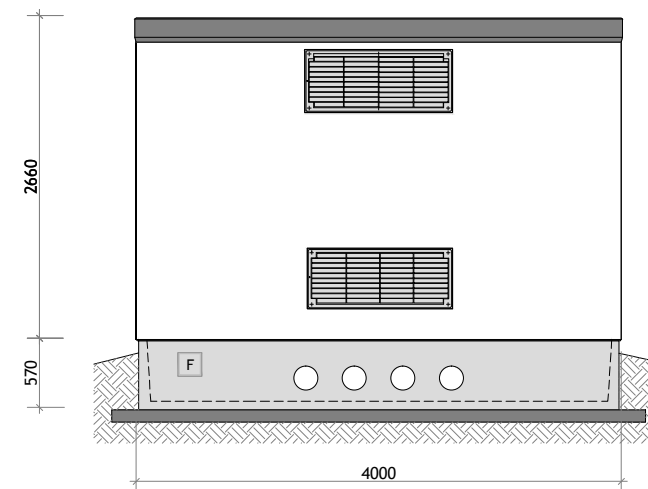
PROSPETTO C
