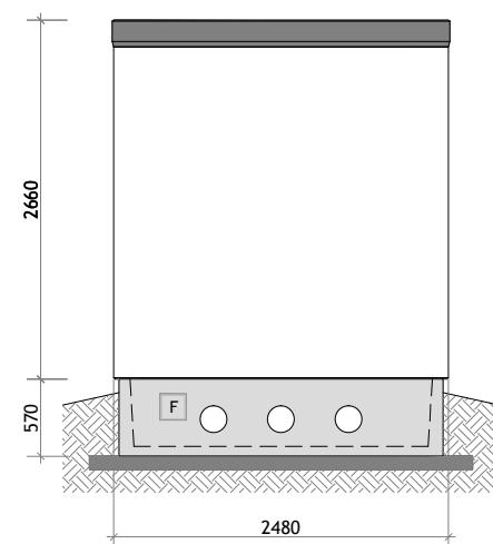
PROSPETTO B
