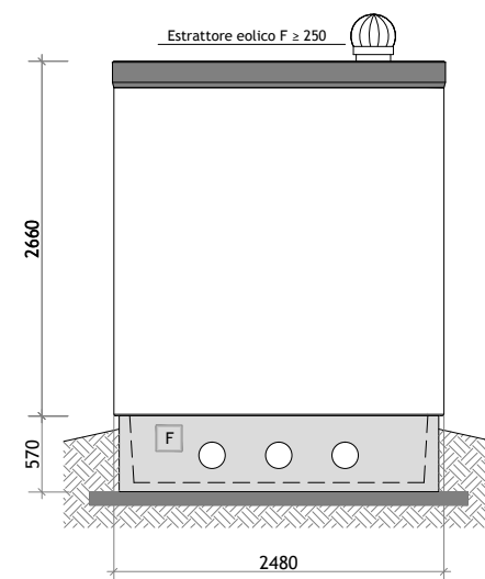
PROSPETTO B
