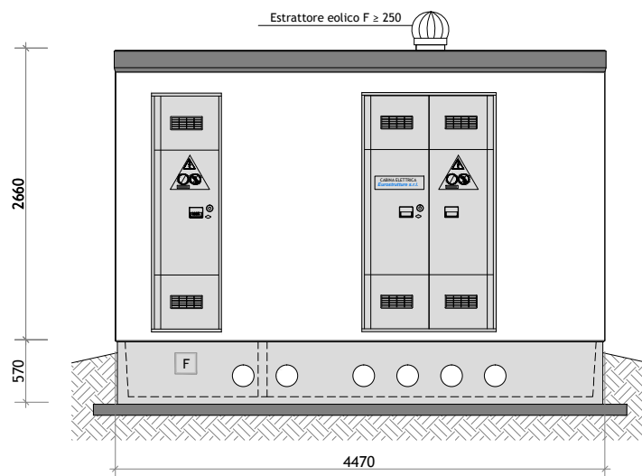
PROSPETTO A
