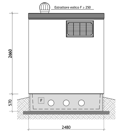
PROSPETTO D
