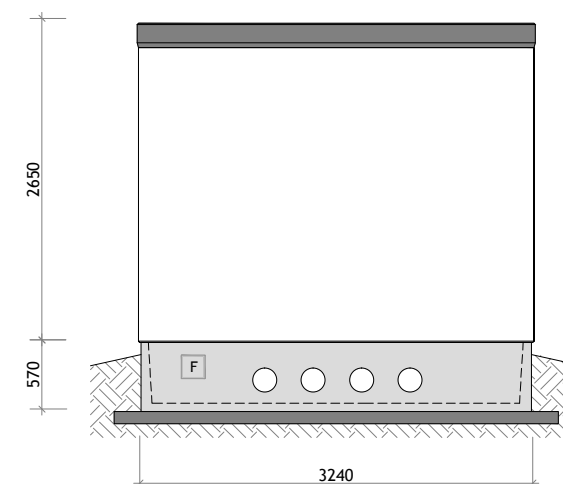
PROSPETTO C
