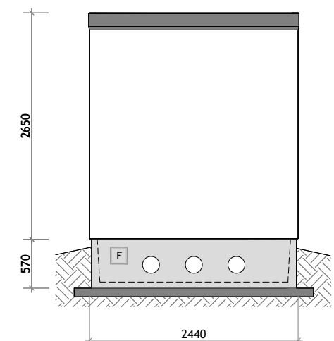
PROSPETTO D
