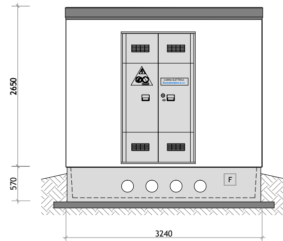
PROSPETTO A
