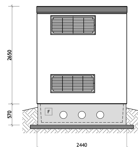
PROSPETTO B
