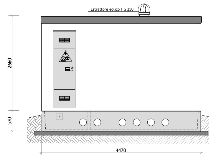
PROSPETTO C
