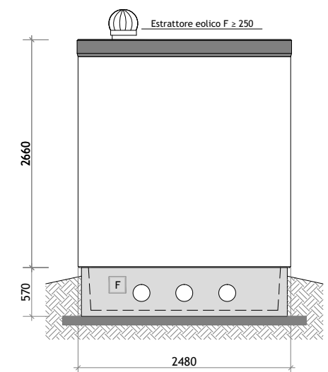
PROSPETTO D
