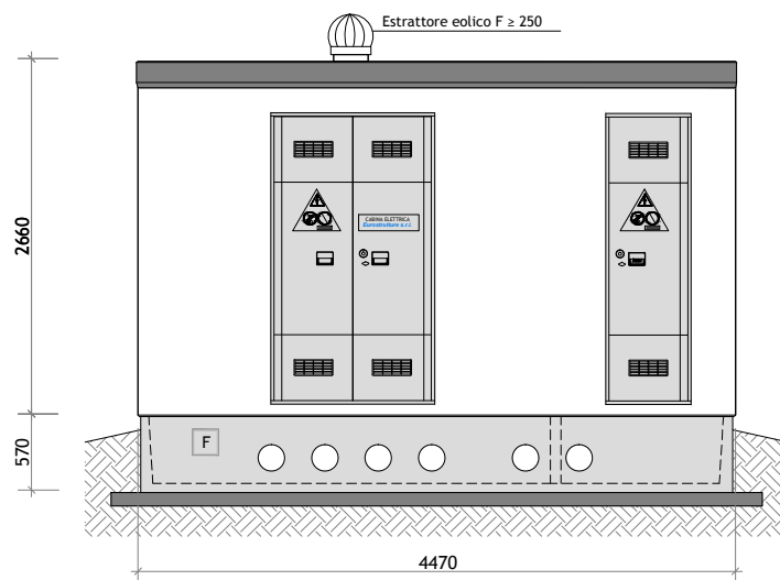
PROSPETTO A
