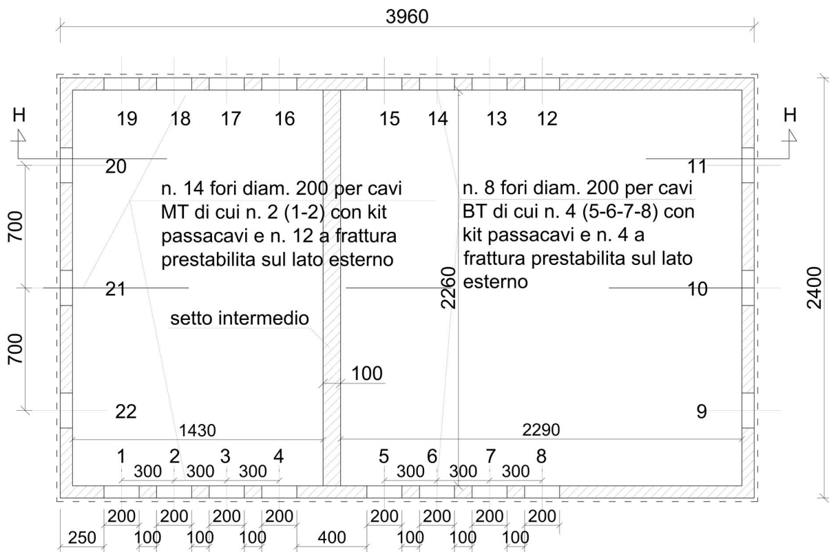
PIANTA BASAMENTO
